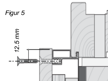
Figur 5: skrue monteres i en avstand av 12,5mm fra aluminiumskant
