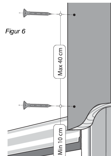
Figur 6: skrue monteres med max 40 cm avstand
